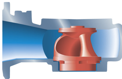
Wirnik kanałowy
